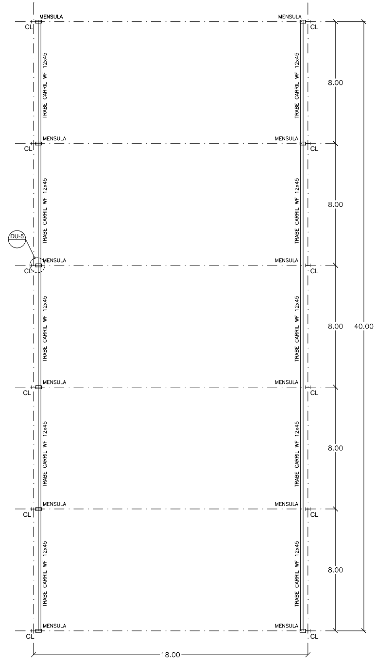
Planta Estructural nivel de Grúa Viajera
