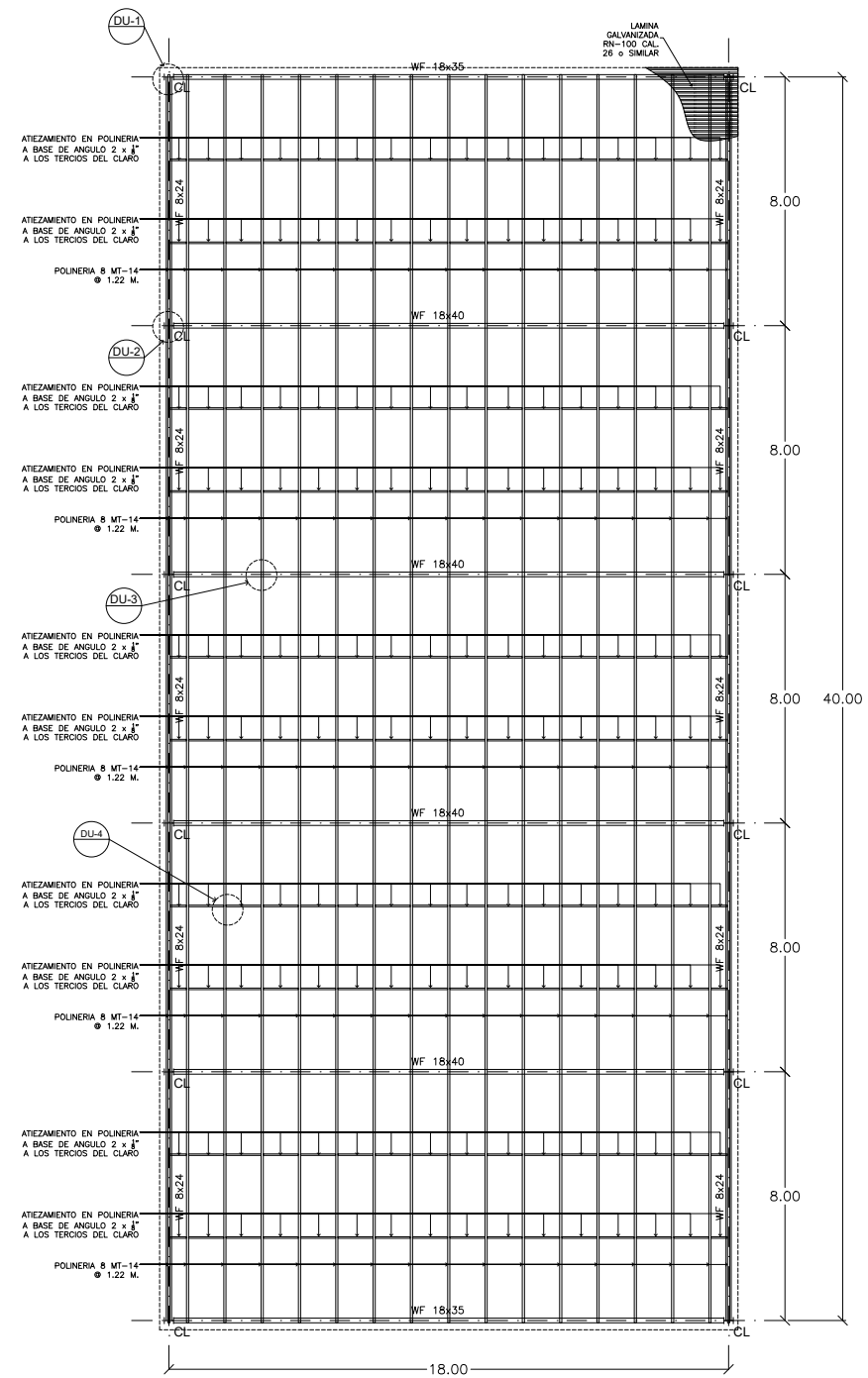
Planta Estructural de Cubierta.
